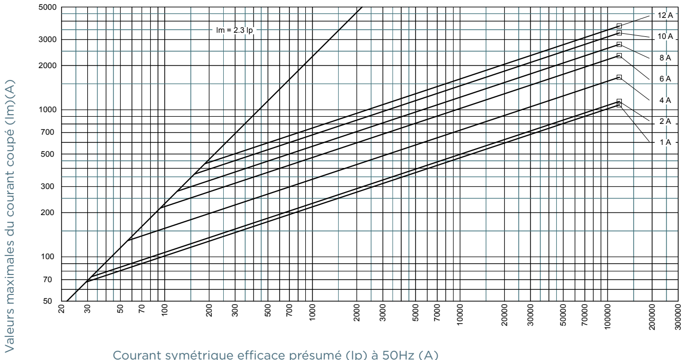
Taille 10x38 400V aM avec percuteur
