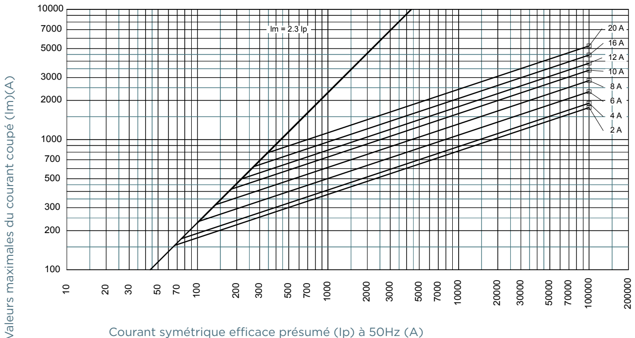
Taille 10x38 400V aM avec percuteur
